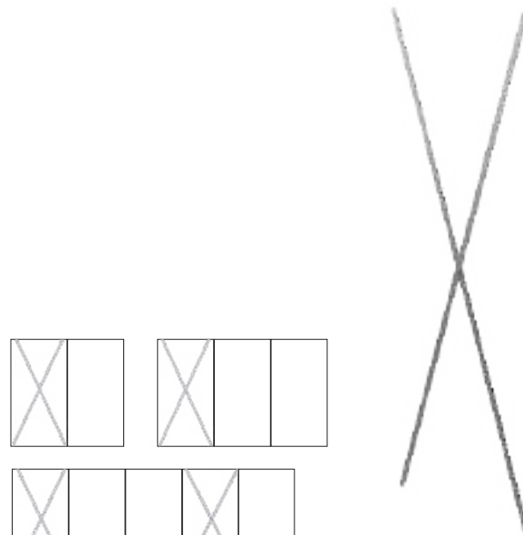
Exemples de disposition des diagonales/panneaux arrière
